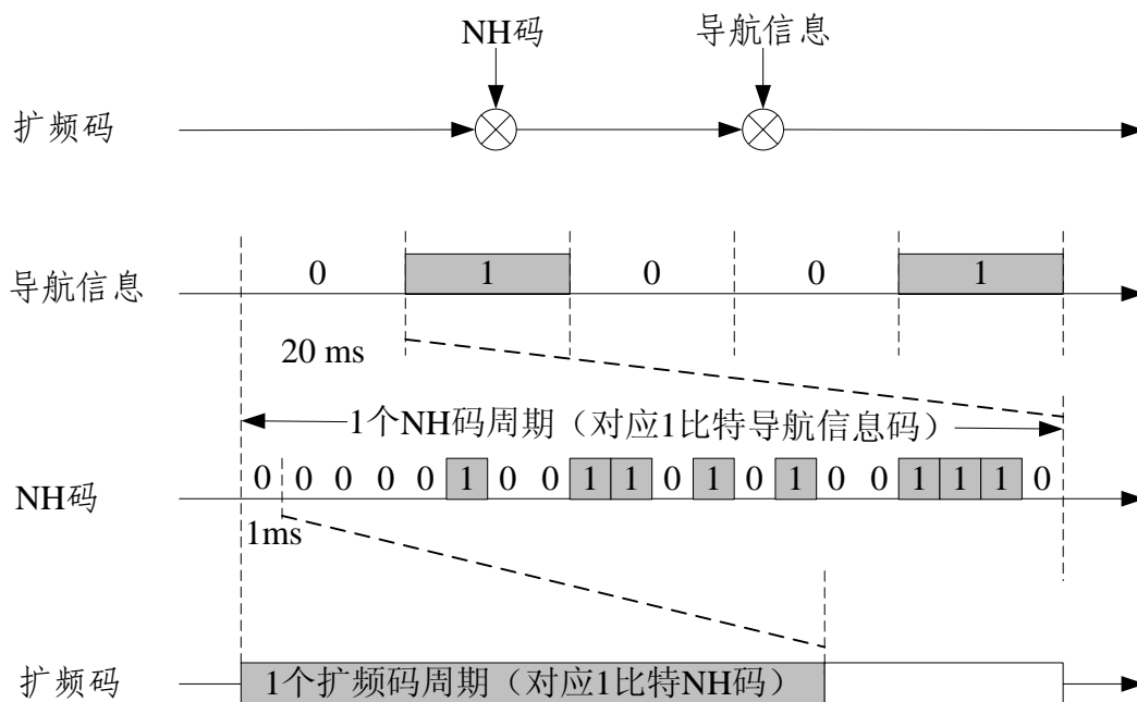
图 5-5 二次编码示意图
