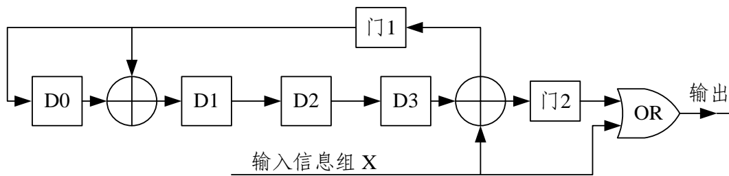
图 5-2 BCH(15,11,1)编码框图
