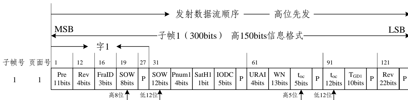
图 5-14-1 D2 导航电文子帧 1 高 150 比特页面 1 信息格式编排
