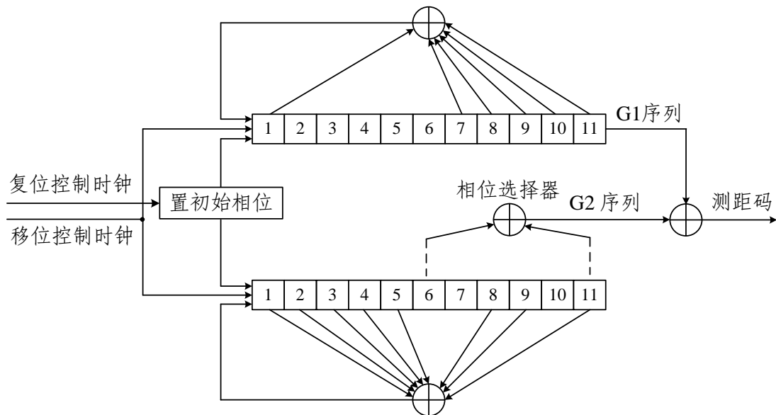
图 4-1 C BII 码发生器示意图
