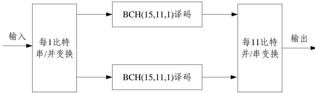
图 5-3 导航电文纠错译码示意图
