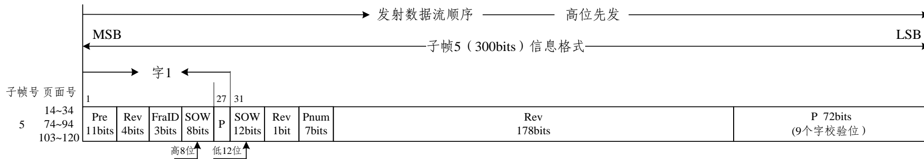
图 5-18-32 D2 导航电文子帧 5 预留页面 14~34，页面 74~94，页面 103~120 信息格式编排
