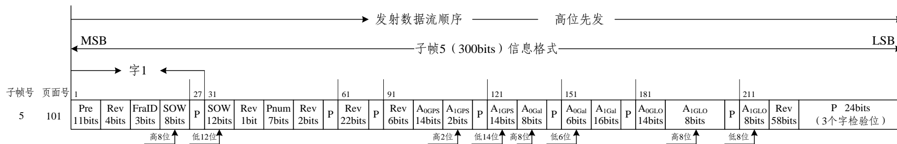
图 5-18-30 D2 导航电文子帧 5 页面 101 信息格式编排
