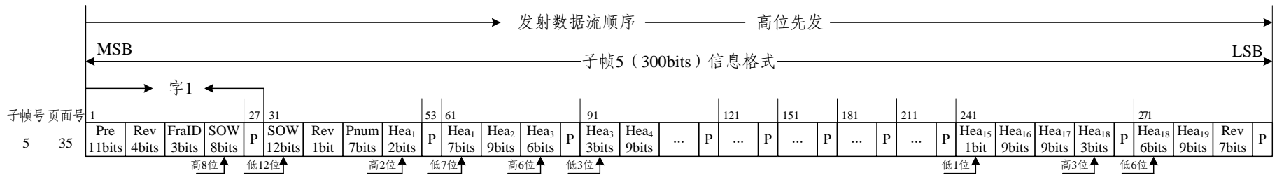
图 5-18-27 D2 导航电文子帧 5 页面 35 信息格式编排
