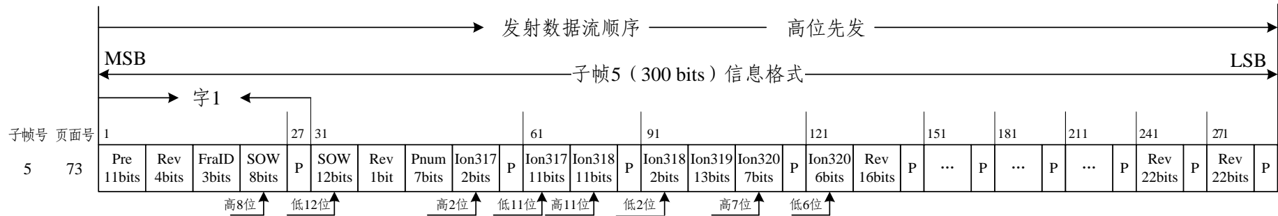
图 5-18-26 D2 导航电文子帧 5 页面 73 信息格式编排
