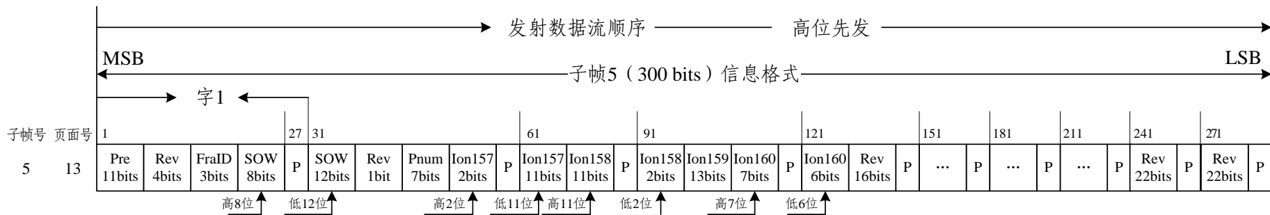
图 5-18-25 D2 导航电文子帧 5 页面 13 信息格式编排
