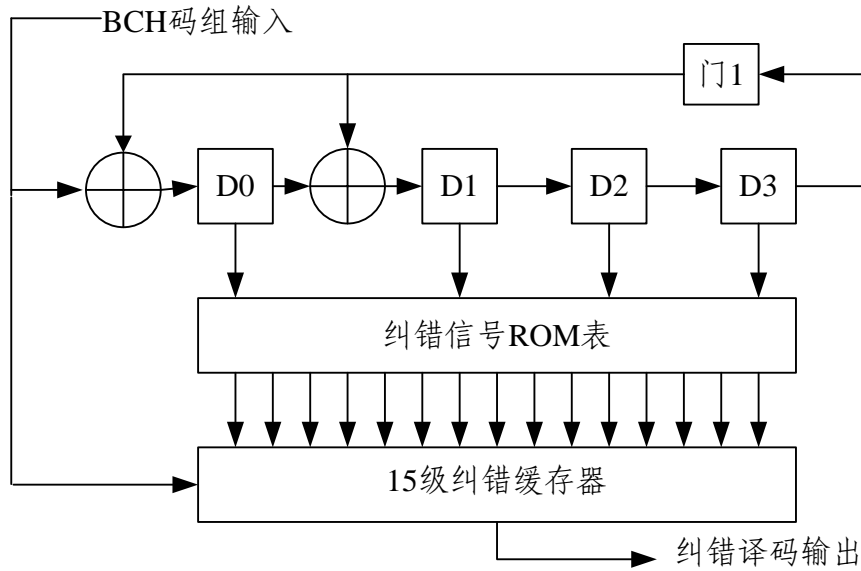
图 5-4 BCH(15,11,1)译码框图
