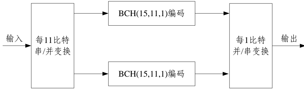
图 5-1 导航电文纠错编码示意图
