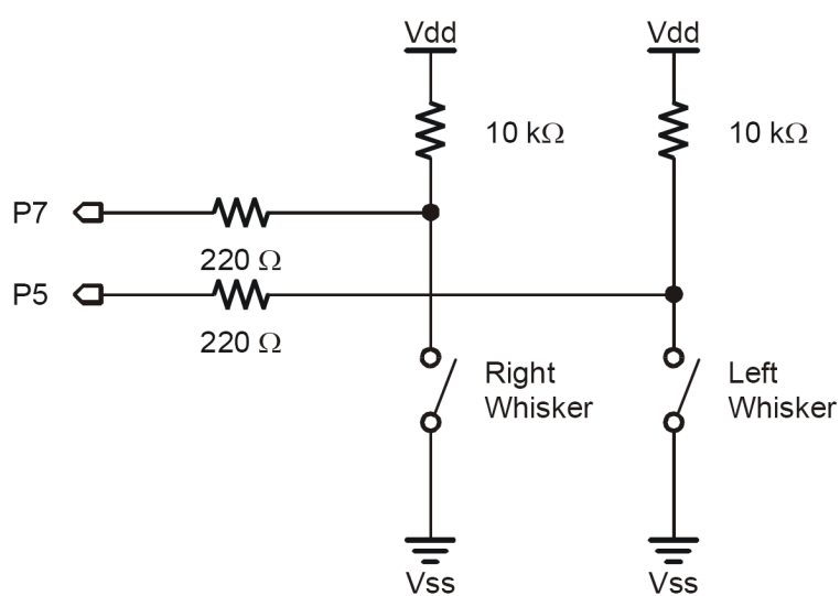
觸鬚電路圖
